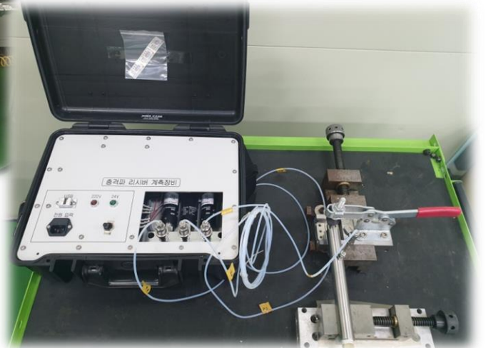
충격파리시버계측시험
