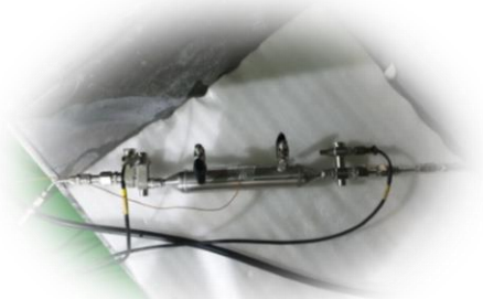
고온작동시험
